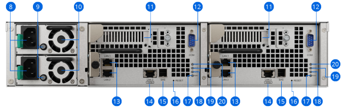
后面板
