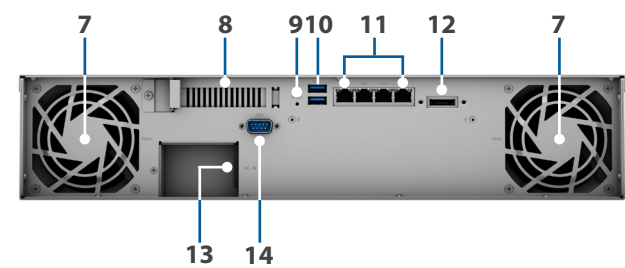
后面板
